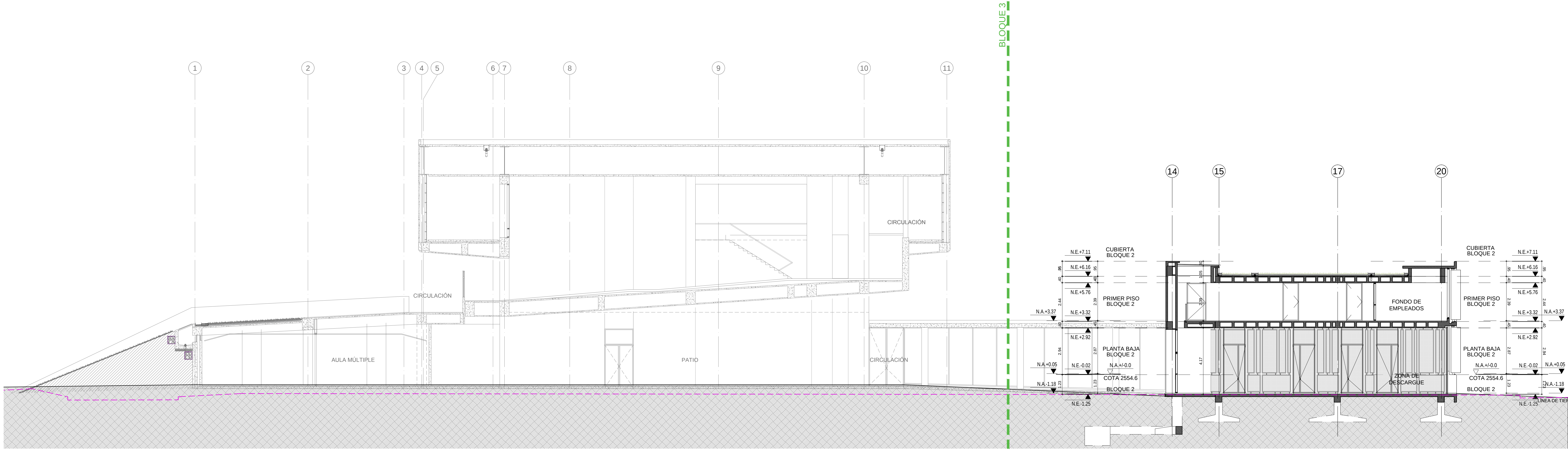
CORTE A - A ESC. 1 : 100
